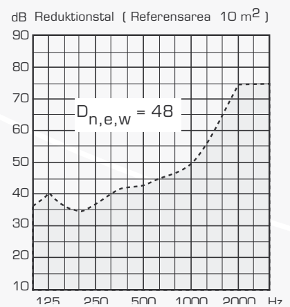
Fresh 90-dB med 400 mm genomföring.
