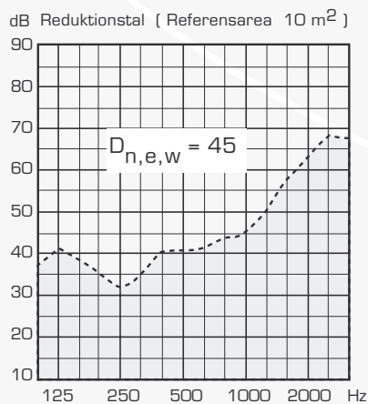
Fresh 90-dB med 300 mm genomföring.
