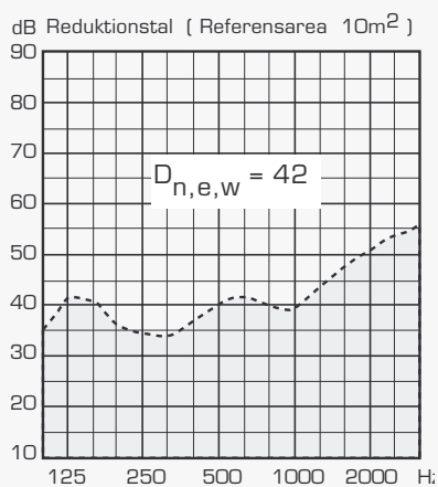
Fresh 90-dB med 200 mm genomföring.
